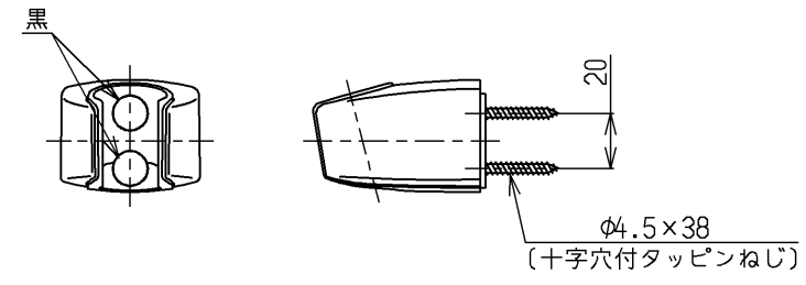
シャワーハンガー(2ヶ)
