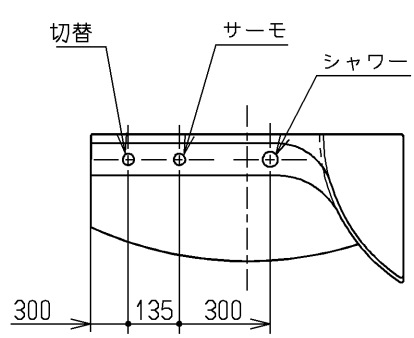
水栓取付け位置 (フリー)
